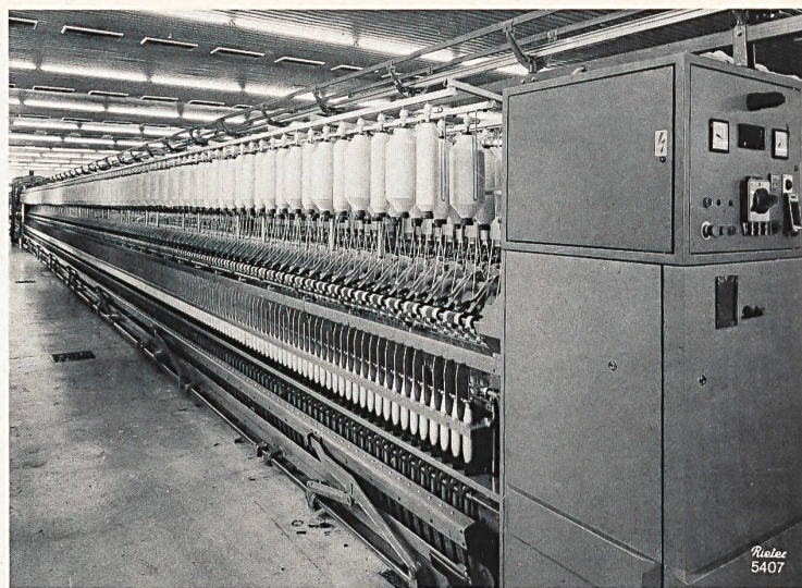
Zu den Selbstverständlichkeiten in der Spinnerei zählt ein moderner Maschinenpark. Dazu gehören beispielsweise Ringspinnmaschinen mit integriertem Doffer und automatischer Hülsenführung (Bild: neuentwickelter Typ G 5/1 von Rieter).
