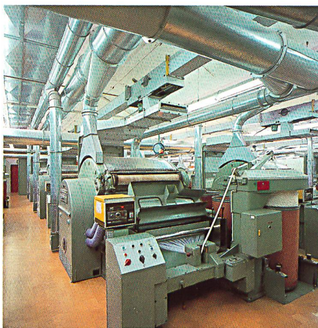
Rieter Aerofeed-F Kardenanlage / La carde Rieter Aerofeed-F / The Rieter Aerofeed-F carding machine.
