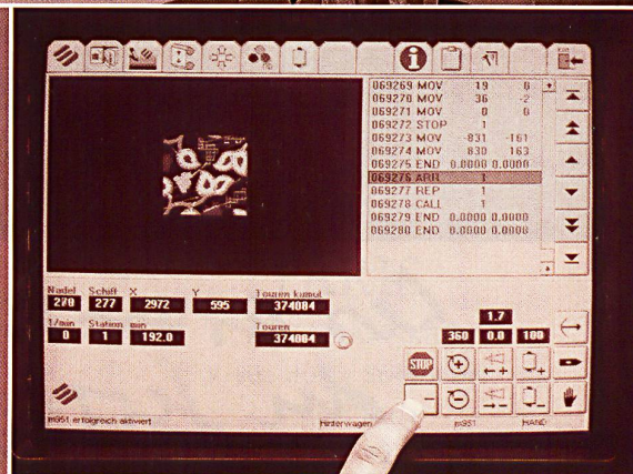
Grafische Benutzeroberfläche «TipControl» mit «Touch-Screen».
