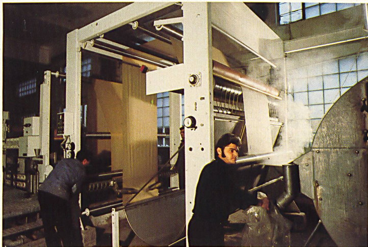
4 Ausschnitt aus der Bleicherei / Vue partielle du blanchiment / Section of the bleaching department.
