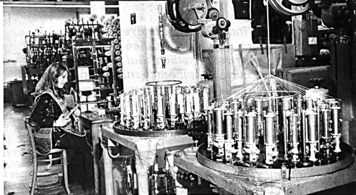
▷ Auf der Flechtmaschine werden Schleuderstäbe, aber auch dickere Kordeln überkloppelt / Sling bars as well as thicker cords are braided on the braiding machine.
