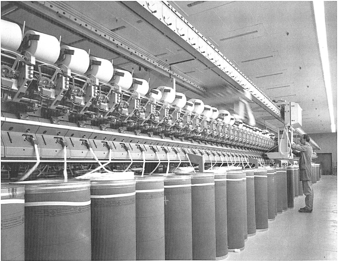
Vollautomatische Hochspinnmaschine
