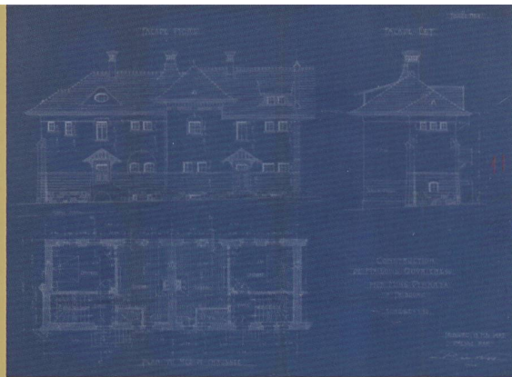
PROJET DE 4 MAISONS OUVRIÈRES CONTIGÜES, DEMI-PLAN DU REZ-DE-CHAUSSÉE, FAÇADE D'ENTRÉE L'ARTICULATION ET PIGNON EST, DEMI-PLAN DU 1 ER ÉTAGE ET FAÇADE SUD AVEC LUCARNE-PIGNON À L'ARTICULATION ET PIGNON EST, FAÇADE SUD AVEC LUCARNE-PIGNON À L'ARTICULATION ET PIGNON EST, CASERNES LOCATIVES ET UNE RÉPONSE À LA CRISE DU LOGEMENT À FRIBOURG, OÙ LE 90% DES APPARTEMENTS COMPTAIENT QU'UNE À DEUX PIÈCES AVEC UN TRISTE RECORD NATIONAL DE 2,67 HABITANT PAR PIÈCE 15 MAI 1907 (EDIL)
