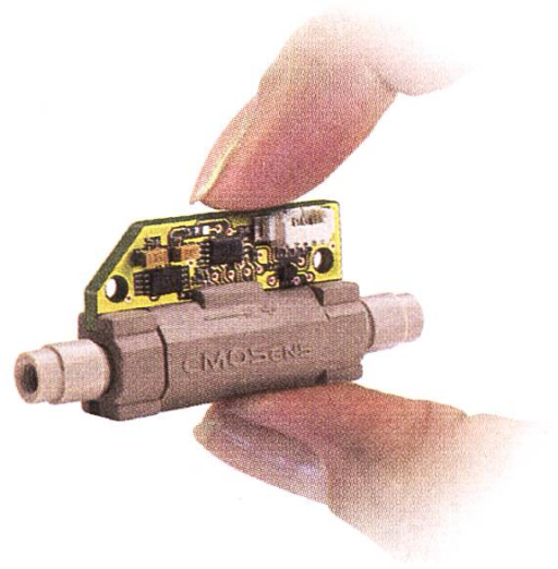
Liquid Flow Sensor LG16 für die medizinischen Diagnostik. Auflösung: 0.5 Nanoliter/Minute
