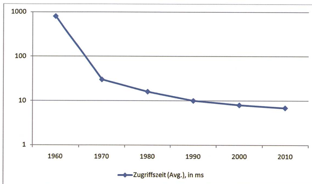
Abbildung 1: Entwicklung der Festplattenzugriffszeiten, logarithmisch
