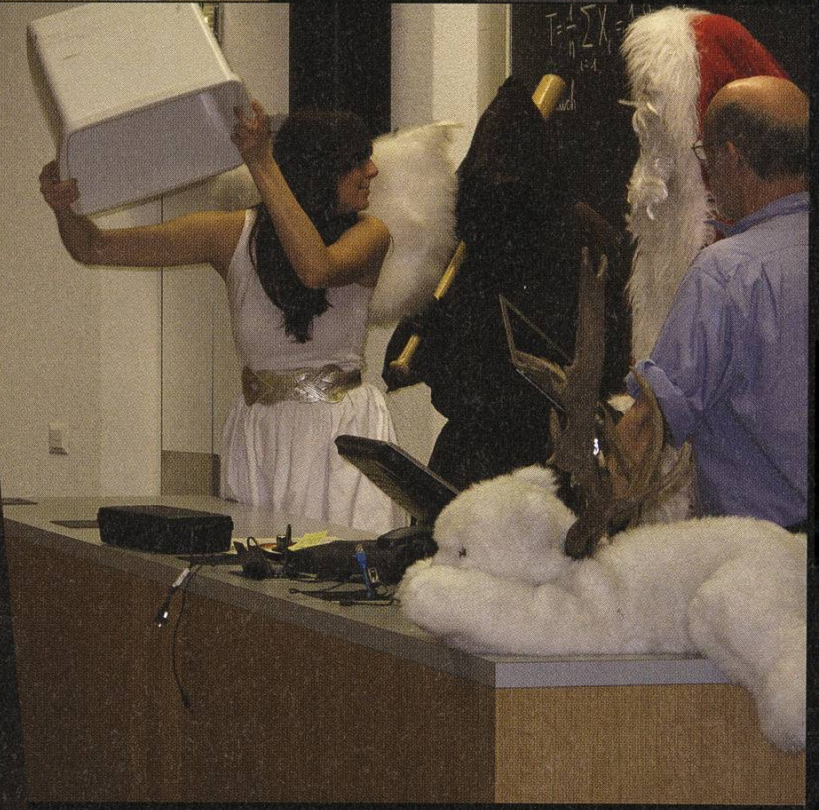
3. Semester: Wahrscheinlichkeit und Statistik, Martin Schweizer
