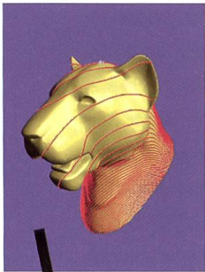
Mesh Parametrization
