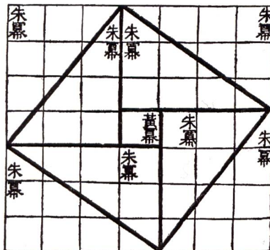
Geometrischer Beweis des Gougu-Theorems im Zhou Bi Suan Jing
