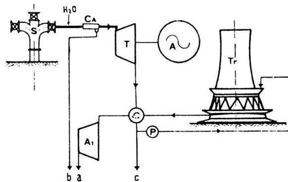
Fig. 5: Condensing geothermal plant, Larderello (ENEL, 1970).
