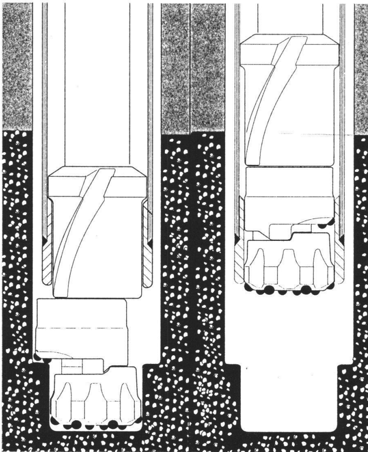
Fig. 1: Beim Ziehen der Hammerkronen wird der Räumers über eine Drehung eingeklappt
