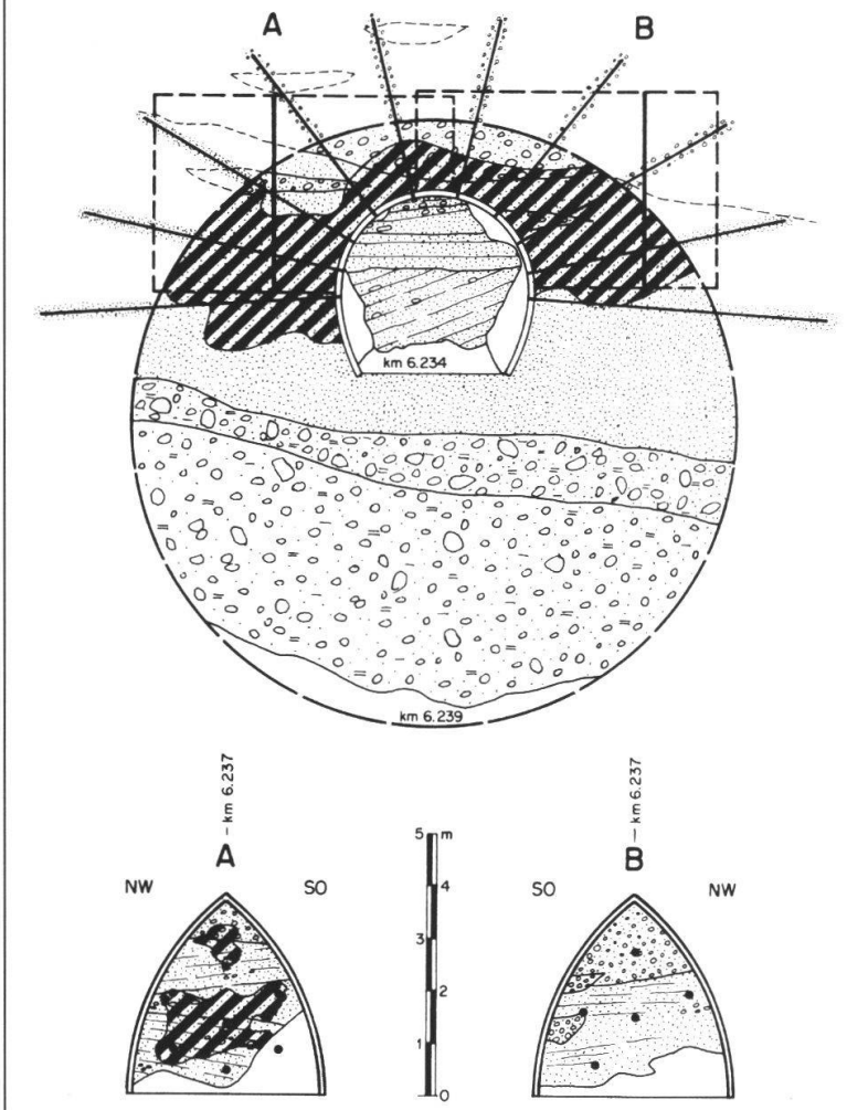
Fig. 7: Geologischer Befund im Bereich der Injektionsversuche aus dem Vorstollen der Weströhre. Die Injektionsbereiche der Vorversuche (km 6.237) wurden in quer zur Vortriebsrichtung stehenden Stollen ausgegraben und die injizierten Bereiche (schraffiert) je Injektionsmittel beurteilt (Brustbilder in den Positionen A und B); nach Ausführung der Hauptinjektionen wurden beim nachfolgenden Schildvortrieb die Geologie und das Ausmass der Injektionen im Ausbruchquerschnitt aufgenommen.
