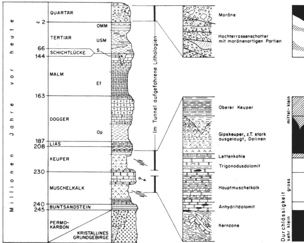
Fig. 2: Gliederung des Schichtstosses im Bereich der Habsburgstruktur mit Angabe der im Tunnel aufgefahrene Abschnitte (OMM: Obere Meeresmolasse, USM: Untere Süsswassermolasse, S: Siderolithikum, Ef: Effinger Schichten, Op: Opalinuston). Der obere Muschelkalk fungiert bei der Therme Bad Schinznach als Thermalwasserleiter; die Evaporite des mittleren Muschelkalks und des Keupers dienten als Abscherungshorizonte bei der Jurafaltung.
