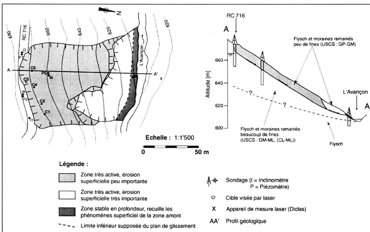
Fig. 1: Carte et coupe schématique du glissement (d'après Maric, 1999).
