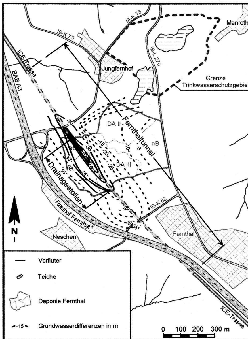
Fig. 8: Grundwasserdifferenzenplan für den Zeitraum November/Dezember 1998 (vor Beginn der Vortriebsarbeiten) und August 2000 (nach Abschluss der Vortriebsarbeiten).
