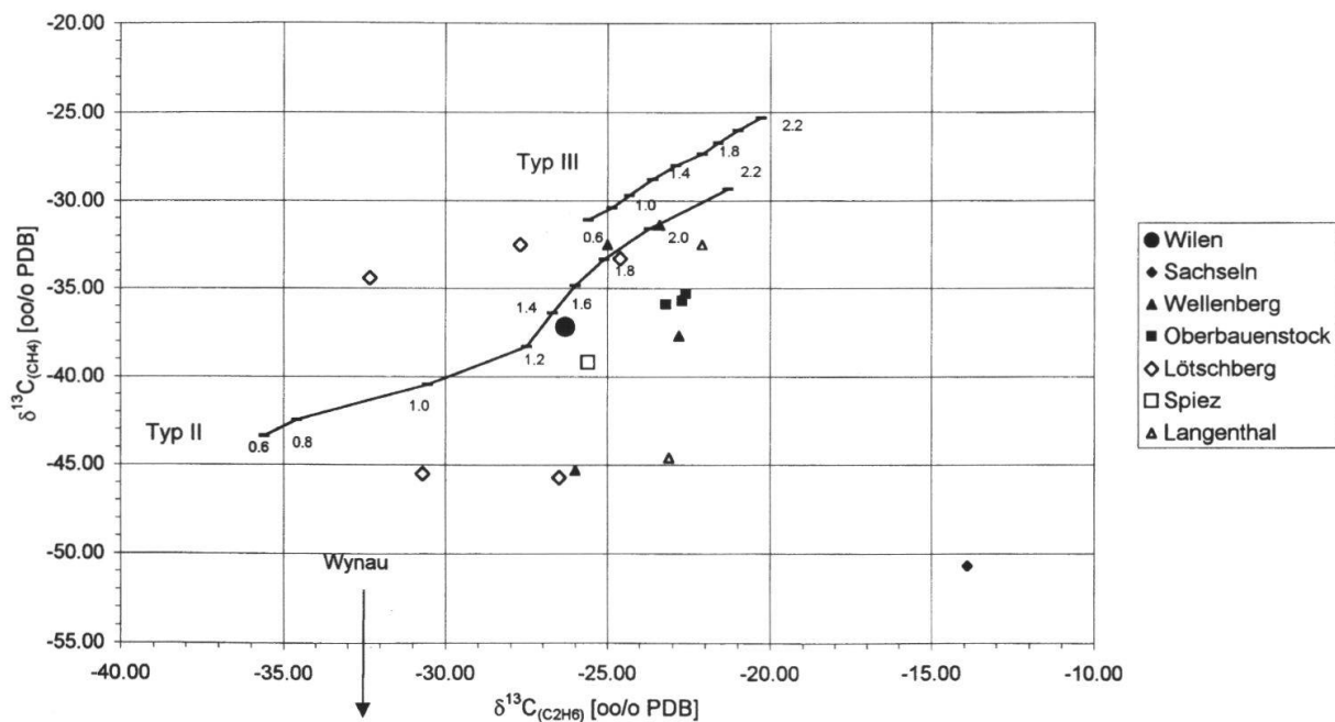
Fig. 9: \delta^{13}C_{(C_2H_6)} - \delta^{13}C_{(CH_4)} -Diagramm nach Berner & Faber (1997): Unterscheidung zwischen verschiedenen Muttergesteinstypen und Abschätzung der thermischen Reife des Muttergesteins aufgrund von Methan- und Ethan-Kohlenstoffisotopen.
