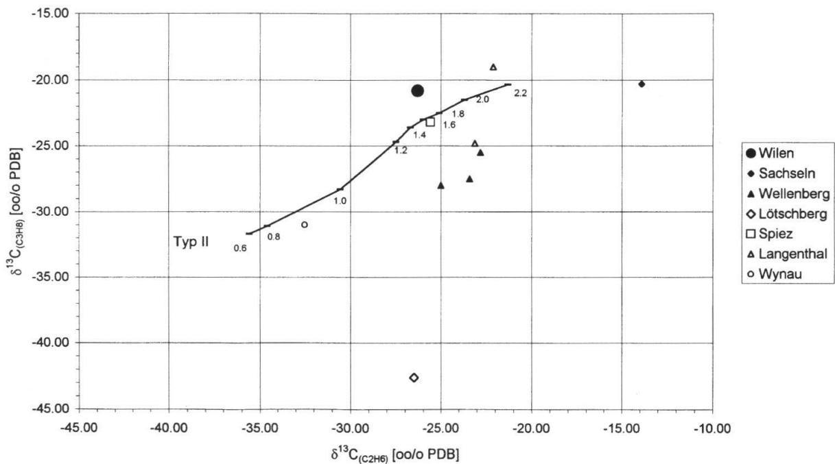
Fig. 10: \delta^{13}\text{C}_{(\text{C}_3\text{H}_8)} - \delta^{13}\text{C}_{(\text{C}_2\text{H}_6)} - Diagramm nach Berner & Faber (1997): Abschätzung der thermischen Reife des Muttergesteins Typ II aufgrund von Ethan- und Propan-Kohlenstoffisotopen.
