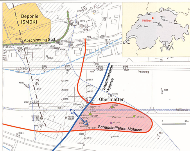
Fig. 8: Lageplan mit Deponie und Schadstofffahne im Molassefeld. Blau schraffiert: Rinnensandstein Ost; rote Fläche: Fahne ausserhalb Zustrombereich Abschirmung Süd; grüne Bohrungen: Pumpbrunnen für Pumpversuche; violette Bohrungen: Impfstellen beim Tracerversuch.
