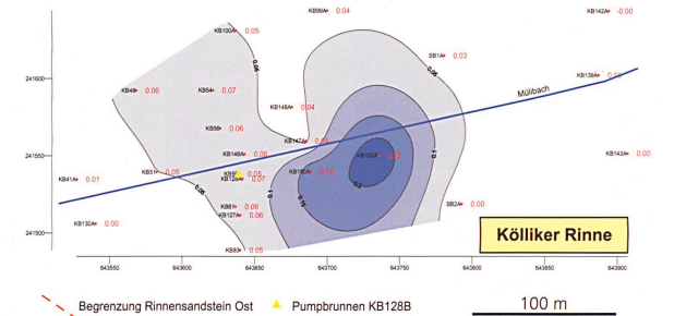
Fig. 13: Absenkrichter in der Molasse [Rinnensandstein Ost] und im Lockergestein der Kölliker Rinne nach 300h Pumpbetrieb in KB128B [Brunnen im Rinnensandstein mit Q=12 \text{ l/min} ]. Die Darstellung erfolgt mittels Isolinen und Messwerten, welche die Potenzialreduktion in [m] darstellen. Massstab: CH-Koordinatennetz.
