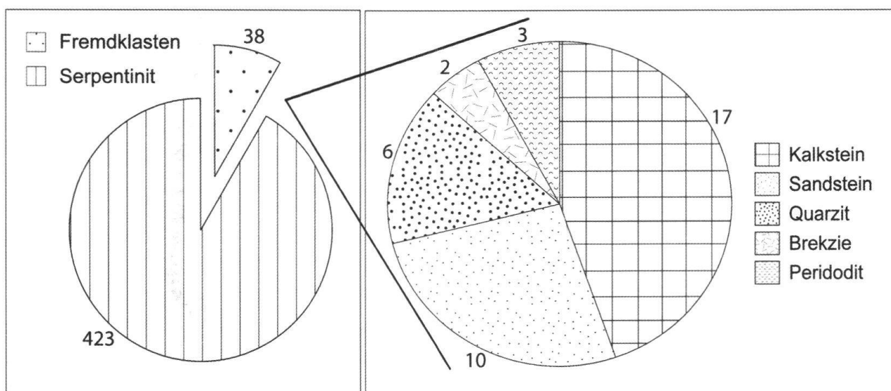
Fig. 8: Anteile verschiedener Lithologien an der Gesamtmenge ausgezählter Klasten.
