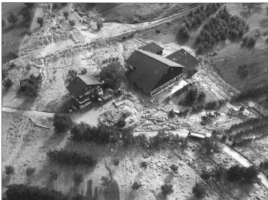
Fig. 8: Übermurtung der SBB-Linie Zug-Goldau und der Liegenschaft Gantlihof in Oberarth am 22. August 2005 (Foto: Kapo Schwyz).
