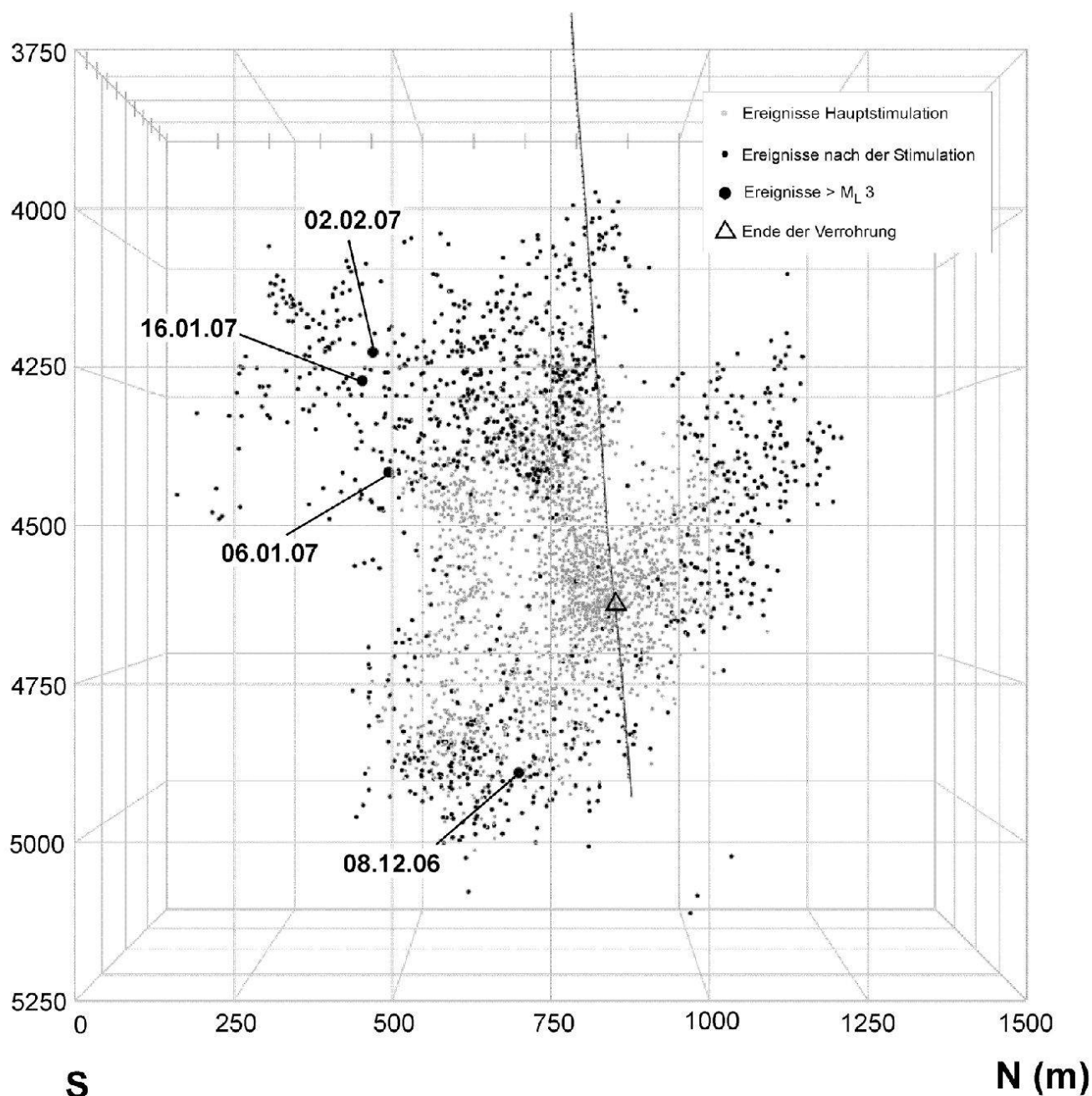
Fig. 8: Seitenansicht des Reservoir Basel 1. Das Dreieck markiert das Ende der Verrohrung und den Beginn der offenen Bohrstrecke (4638-5000 m). Übrige Parameter wie in Figur 7.
