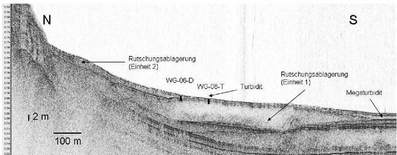
Fig. 11: Seismisches Profil vor Weggis (Profilspur in Fig. 10) mit den beiden Rutschungsablagerungen (Einheit 1 und 2) und den entnommenen Kurzkernen WG-06-D und WG-06-T.
