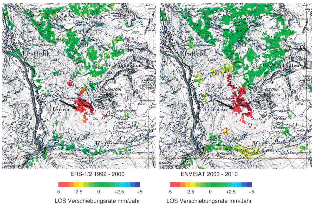
Fig. 5: Mittlere Verschiebungsrate im Gebiet der Chli Windgällen in den Jahren 1992 bis 2000 (Satellit ERS; links) und 2003 bis 2010 (Satellit ENVISAT; rechts). Massstab ca. 1 : 80'000. Der schwarze Pfeil markiert einen Punkt, von dem die Verschiebungsdaten in einer Zeitreihe dargestellt sind (Fig. 6, 7).
