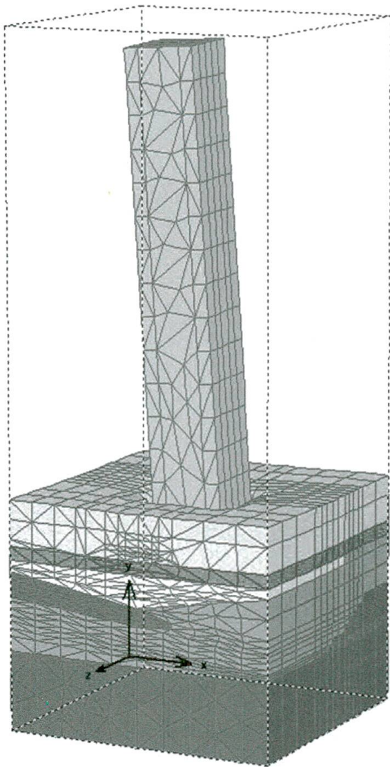
Fig. 5: Città di Castello tower mesh for the FEM analysis.
