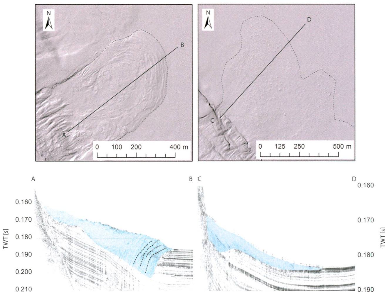
Fig. 5: Morphologie der Fronten (blau) der Oberrieden-Rutschung [1918] (links; Nr. 1 in Fig. 2) und der Horgen-Rutschung [1875] (rechts; Nr. 4 in Fig. 2) mit darunterliegenden 3.5 kHz - Pinger reflexionsseismischen Profilen (Strasser 2008).
