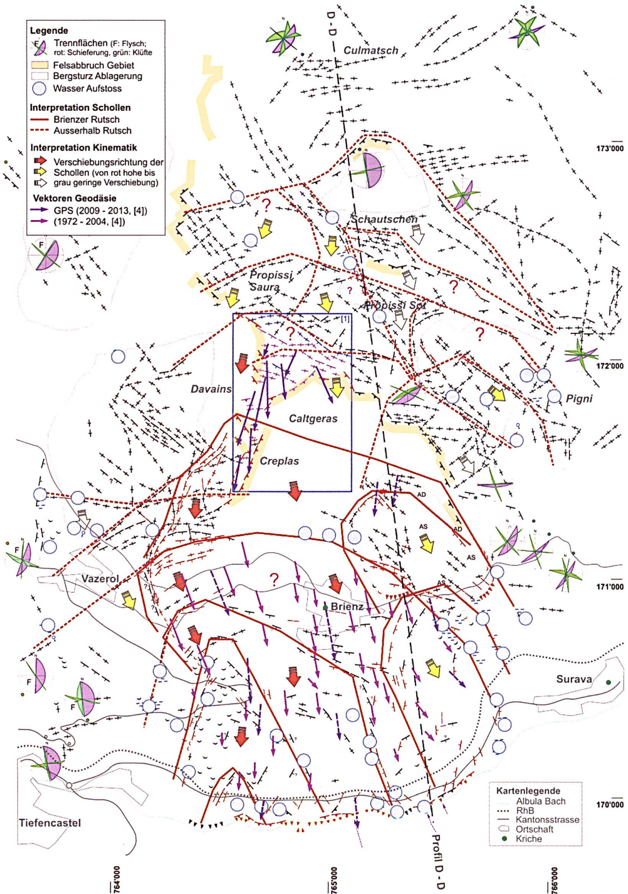
Fig. 7: Abgrenzung von aktiven Schollen des Brienz Rutsch und deren Fortsetzung im Felsgebiet oberhalb. Wasser Aufstösse folgen meist den Schollengrenzen. Entsprechend der kinematischen Freiheitsgrade der einzelnen Schollen sowie der geologischen Disposition wurden ihre Bewegungsrichtungen theoretisch ermittelt (Signaturen Feldaufnahmen gem. Fig. 6).
