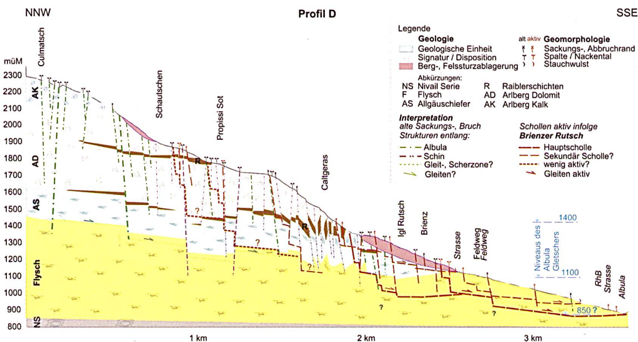
Fig. 10: NNW-SSE verlaufendes, geologisches Profil D mit den mehrere 100 m tief bis in den nach E - SE einfallenden Flysch hinunter reichenden Graben-, Sackungs- und Rutschstrukturen [2].
