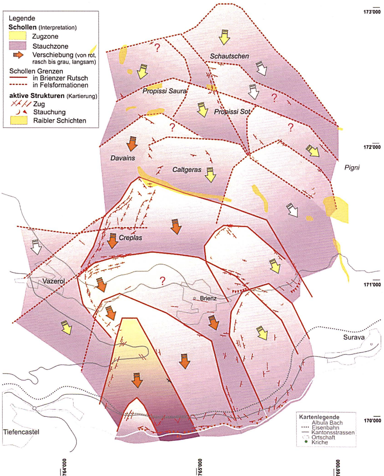
Fig. 9: Kinematische Interaktionen zwischen den talwärts gleitenden Schollen des Brienzer Rutsches mit stets sich verändernden Zug- und Stauchzonen und den «aktiven» Auswirkungen bis in die Felschollen von Propissi und Schautschen auf ~ 1800 m ü.M.
