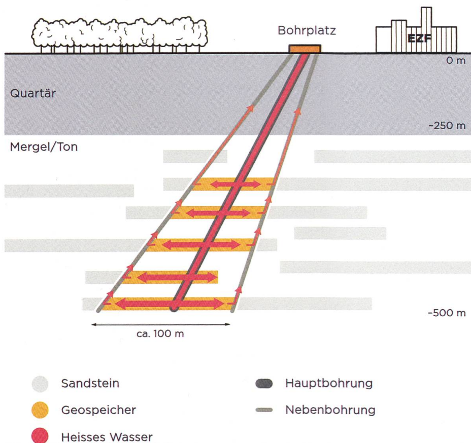
Fig. 1: Schematische Darstellung des Geospeichermodelles für die Untere Süsswassermolasse. Eingezeichnet sind die Hauptbohrung und zwei Nebenbohrungen. Je nach Durchlässigkeit der Sandsteinlagen sind weitere Nebenbohrungen notwendig. Die Pfeile geben die Flussrichtung an [1].
