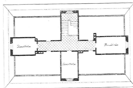
Dachgeschoss
