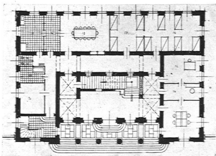
Projet de concours pour un bâtiment de district Le Locle
