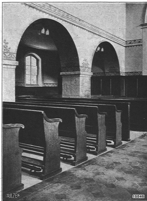
KIRCHE OBERWINTERTHUR, ELEKTR. NIEDERDRUCK- DAMPFHEIZUNG MIT UNTER DEN FUSSSCHEMELN VERLEGTE HEIZROHREN
