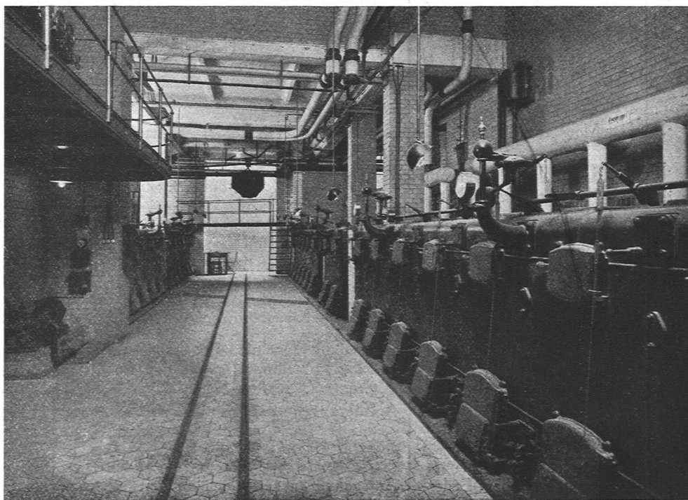
Catenakessel - Anlage, 26 Feuer = 520 qm
