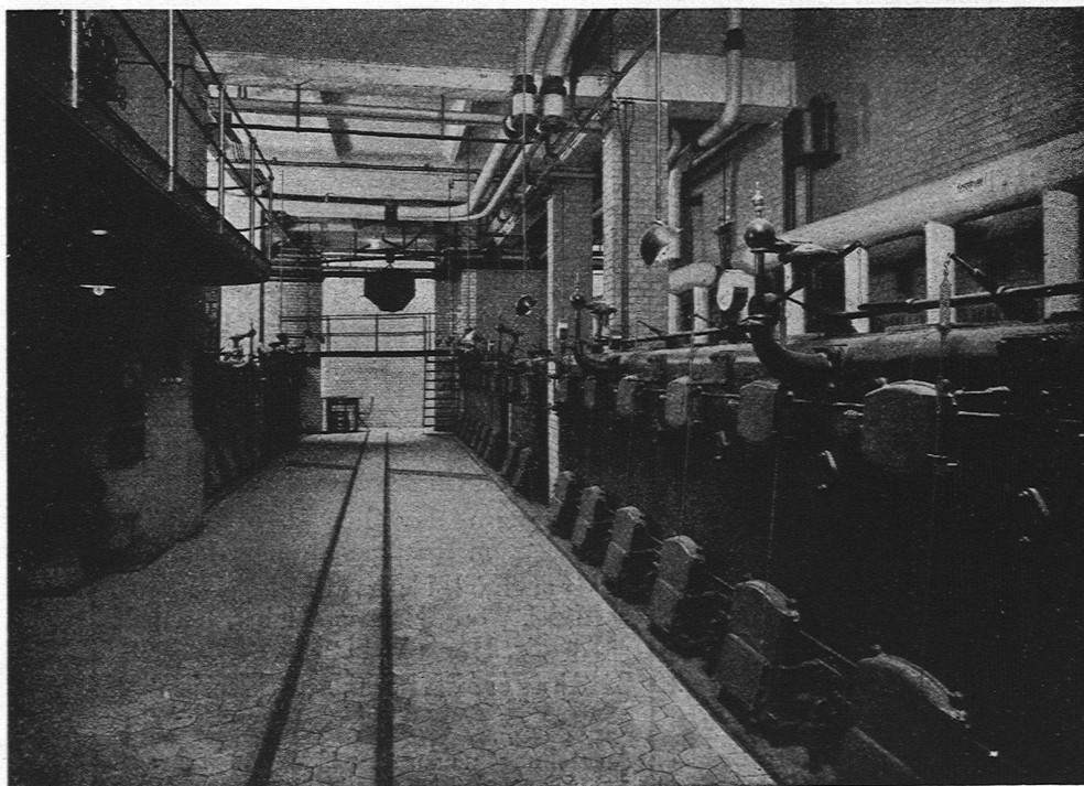
Gatenakessel-Anlage, 26 Feuer = 520 qm
