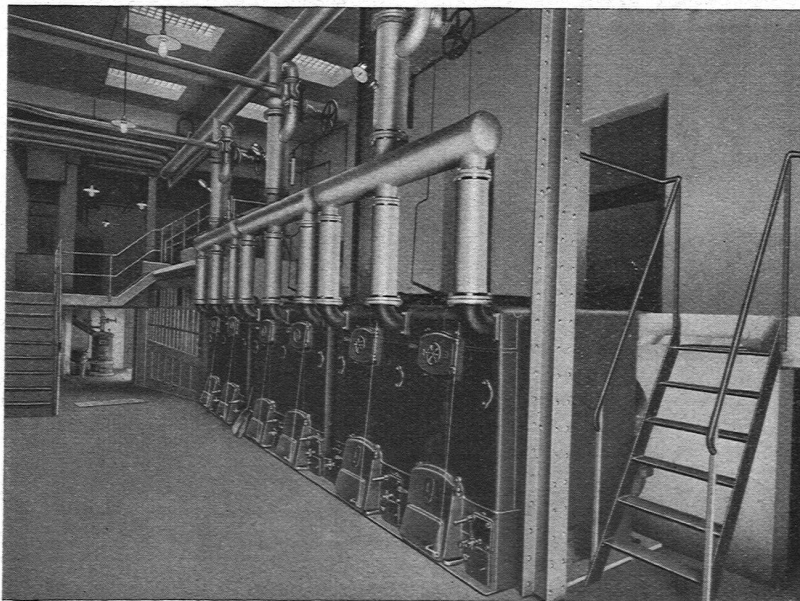
Geschäftshaus Anf. Inst. Orell Füssli, Zürich. Catena-Kessel.
