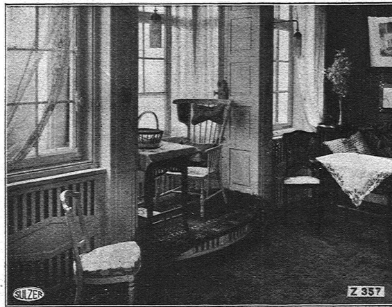
Abb. 12. Heizkörperaufstellung in den Fensternischen und dem Erker eines Wohnzimmers. Der Erkerfussboden wird durch einen Doppelboden und die darunter durchströmende Raumluft warm gehalten.
