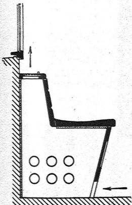
Abb. 13. Schnitt durch eine Erker-Sitzbank mit darunter gelegten Heizrohren.
