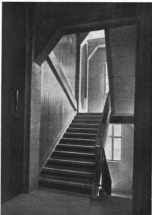
Abb. 2. Patentreppe in der Stickerei Eugster, Altstetten (Rheintal), auf Eisenbeton-Rahmen montiert, als feuersichere Anlage in bestehenden Holzbau eingebaut.
