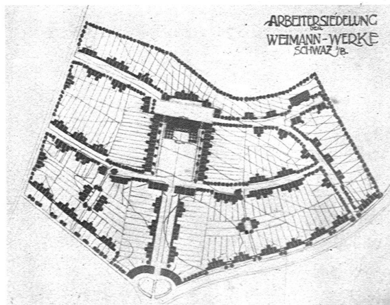
SIEDLUNG SCHWAZ IN BÖHMEN Grundrisse
