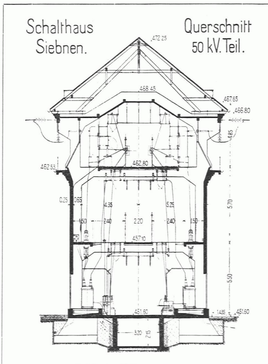
35. ZENTRALE SIEBENEN SCHALHAUS-QUERSCHNITT
