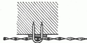
Abb. 4. Befestigung von Rauchs Reformrabit an Holzbalcken.
