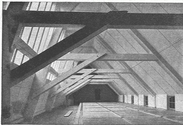
Feuersicherer Ausbau eines Dachstuhles mit Eternit-Platten
