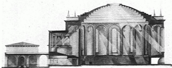
ARBON / SCHNITT
