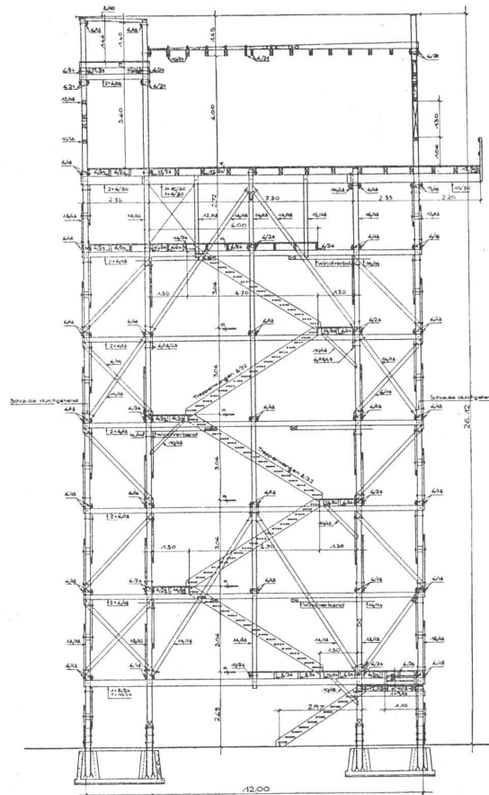
Schnitt B-B.
