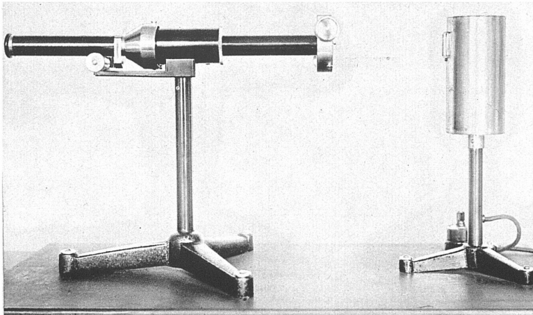
ANOMALOSKOP, Modell IIb Optik und Mechanik A.-G., Basel
