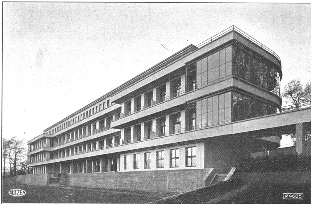
„Lory-Spital“ (Inselspital) in Bern, ausgerüstet mit Sulzer-Pumpen-Warmwasserheizung und Dampfkochküche mit Ventilationsanlage.
