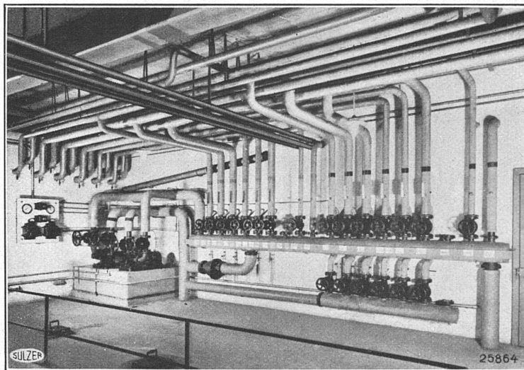
Geschäftshaus „Stampfe“ Zürich. Zirkulationspumpen und Verteiler der Sulzer-Warmwasserheizung.
