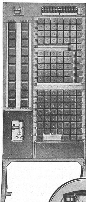
Automatische Haus- zentrale Hasler für 50 Stationen und neuer Telefon- apparat Hasler
