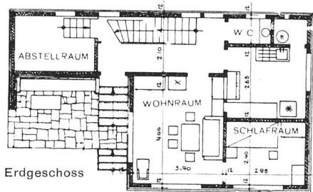
Grundrisse 1:200
