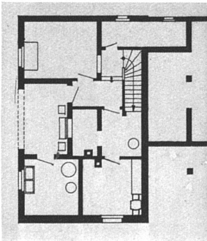
Dachgeschoss- und Kellergeschoss- Grundriss 1:300
