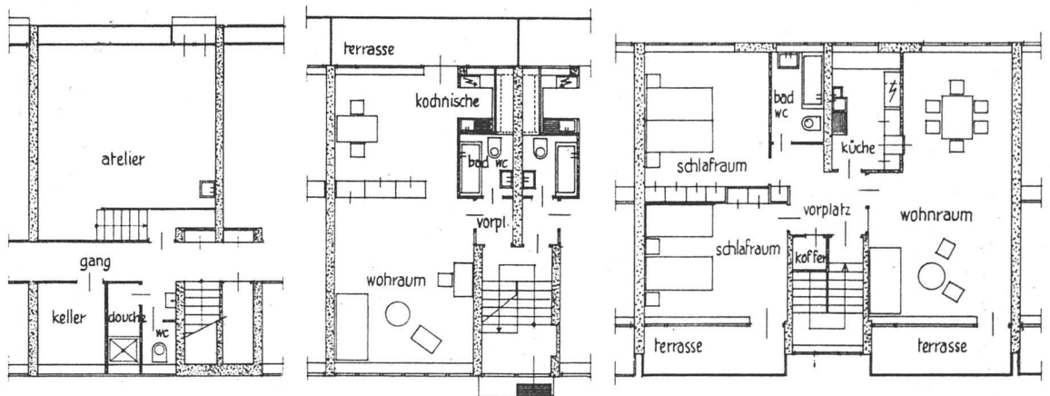
Atelierhaus Typ N Grundrisse 1:200 Die Ateliers im Untergeschoss können separat vermietet werden
