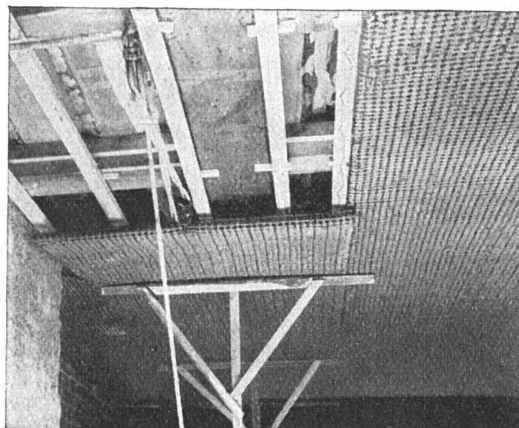
Rissfreie Drahtziegeldecken
