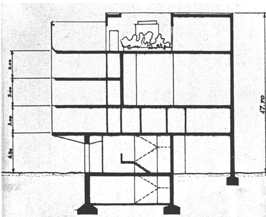
Grundrisse 1 : 300 Schnitt 1 : 400
