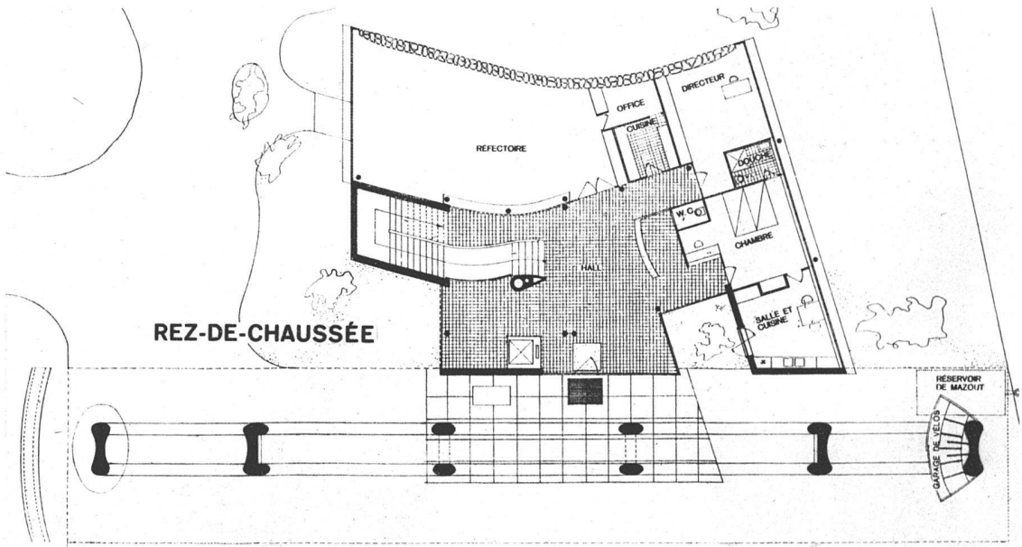
Grundrisse 1 : 300 Schnitt 1 : 400
